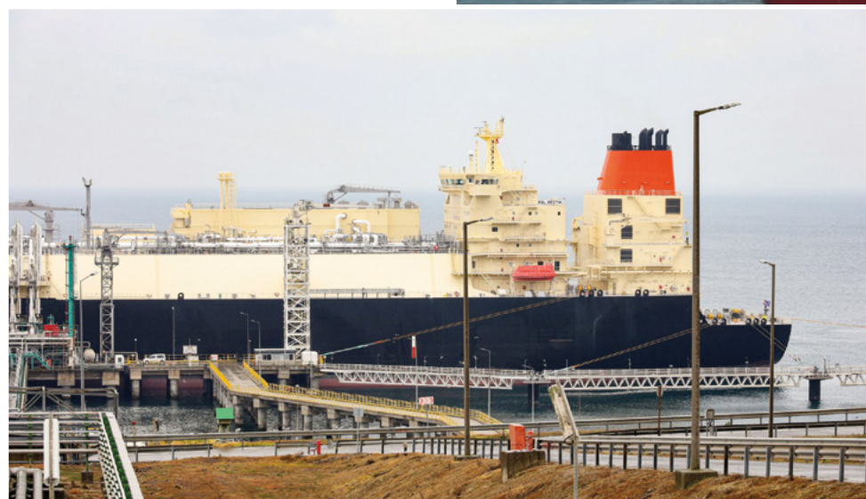
Το LNG terminal Marmara Ereğlisi, εμφανίζεται με send-out προς το σύστημα 37 εκατ. m 3 /ημέρα
